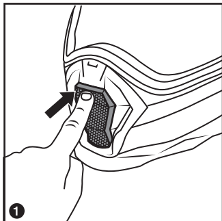
REMOVE THE AIR VENT CAP
